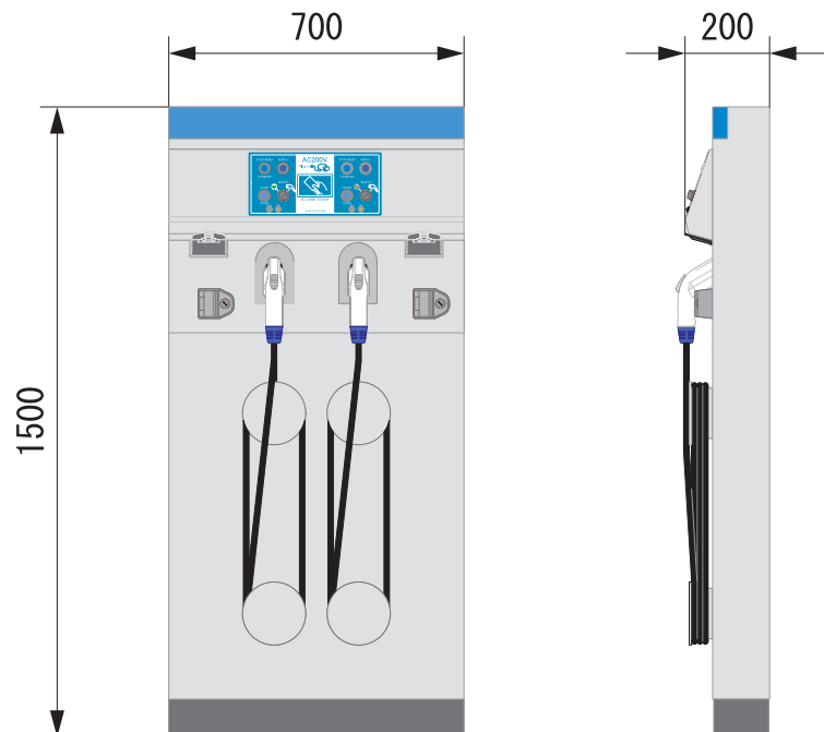
外形寸法図
